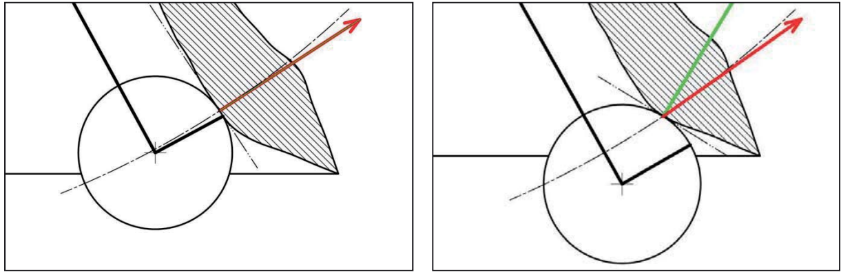
Abbildung 4: Variation der Klöppelanschlagrichtung (Stoßrichtung Pfeil, Flächennormale grau), links: Klöppellänge optimal; rechts: Klöppel zu lang
