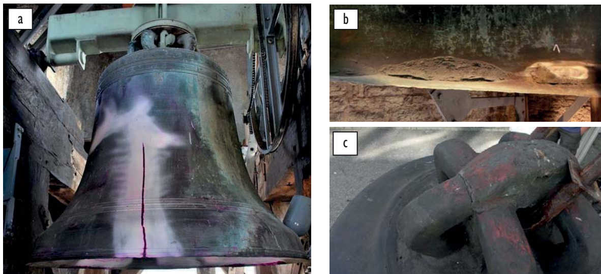
Abbildung 2: Schäden an Glocken: a) Ermüdungsrisse; b) Schlagverschleiß; c) Fertigungsfehler
